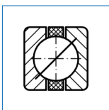
Schrägkugellager PBSD 12,7 x 12,7 mm 1/2"
