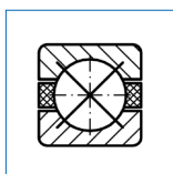
Vierpunkt Axialkugellager PBAD 12,7 x 12,7 mm 1/2"
