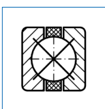
Vierpunktlager PBXD 12,7 x 12,7 mm 1/2"
