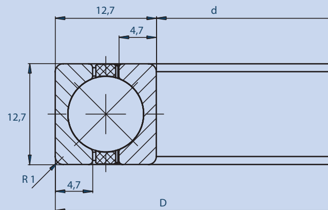
Lagermaße
