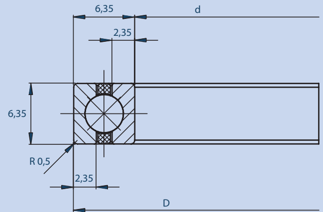
Lagermaße
