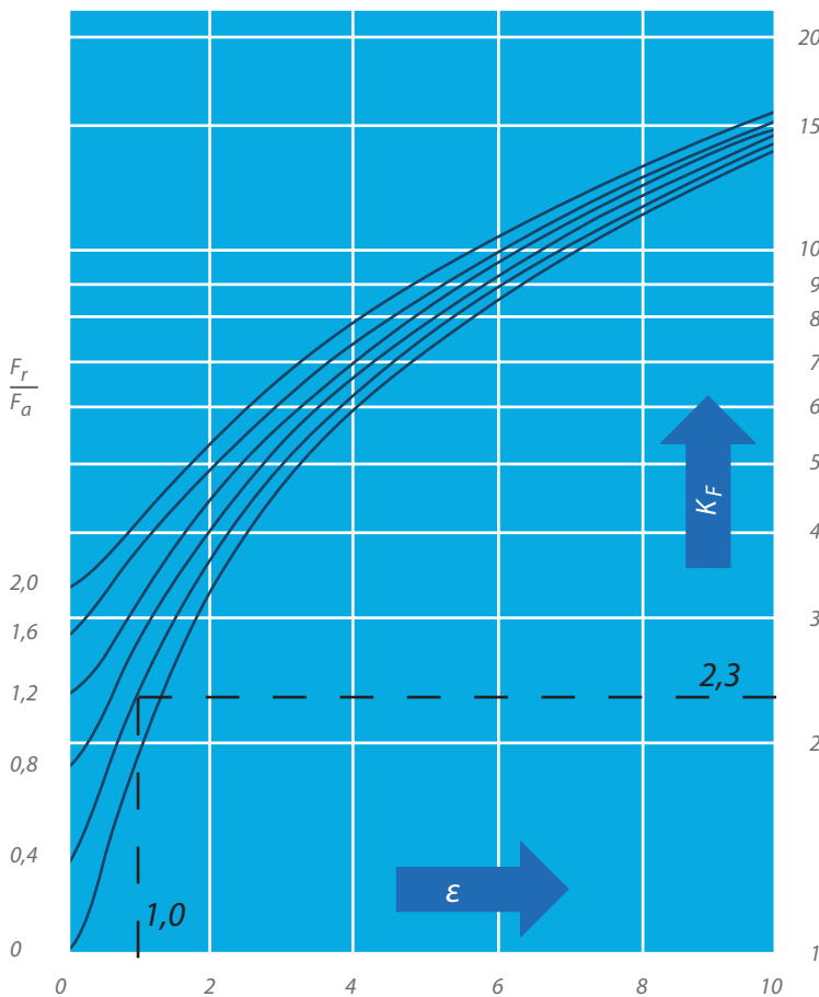
Dyn. Lastfaktor K_F für Vierpunkt-Dünnringlager
