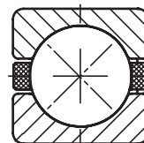
Axialkugellager PBAD 12,7 x 12,7
