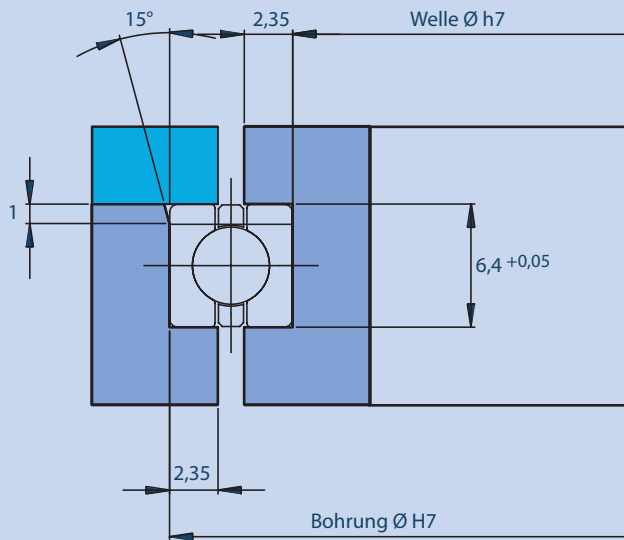
Einbaumaße
