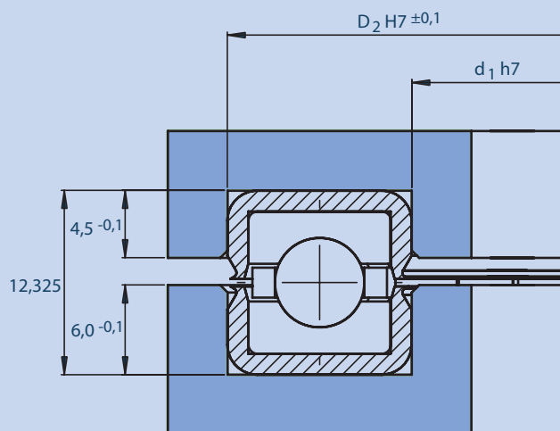
Einbaumaße
