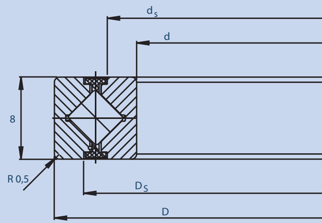
Lagermaße
