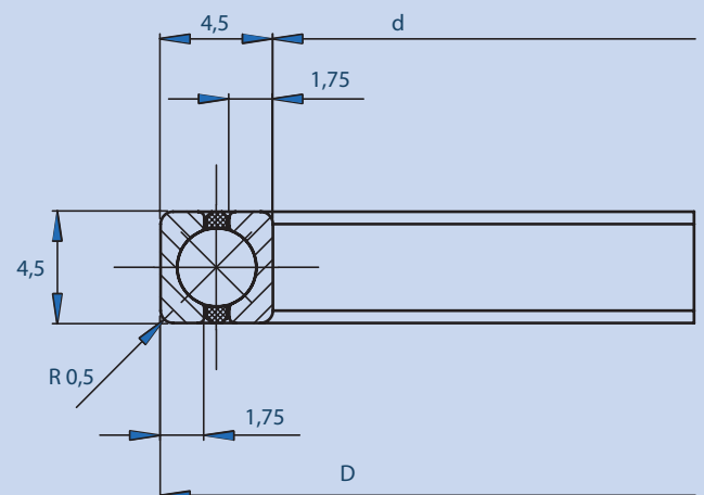
Lagermaße
